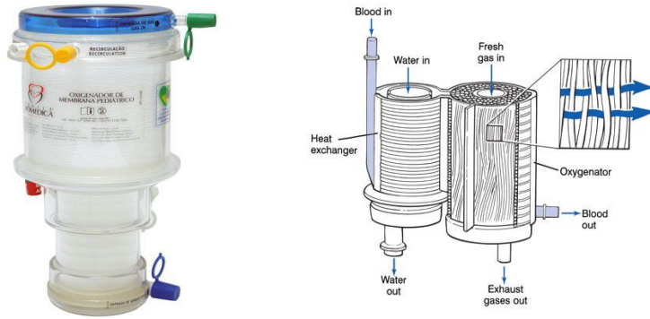
Resim 4.6: Membran Oksijenatör
