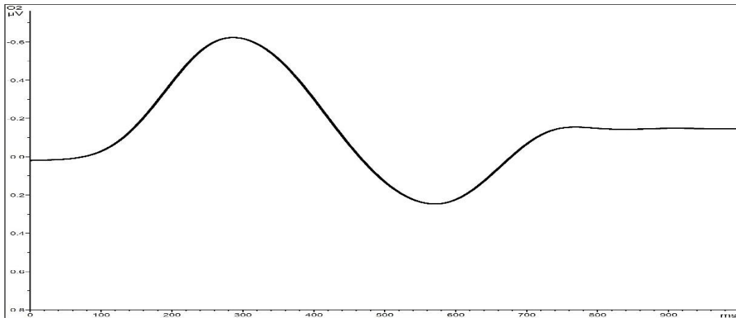
Şekil 4.1. Delta dalgası
