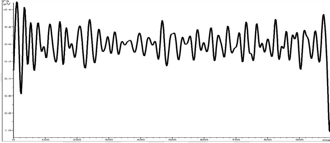
Şekil 4.5. Gama dalgası
