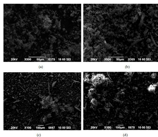
Figure 4. Morphology of \beta -CD complexes containing: (a) 5%; (b) 10%; (c) 15%; and (d) 20 wt % VRCZ.
