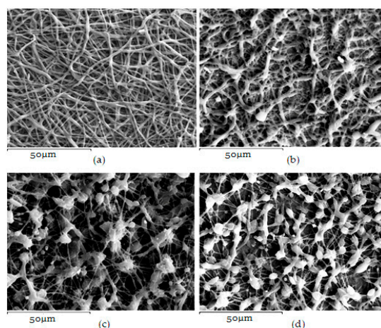
Figure 3. PCL fibers containing: (a) 5%; (b) 10%; (c) 15%; and (d) 20 wt % of Voriconazole (VRCZ) drug.
